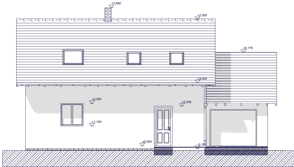
FASADA DO ULICE
